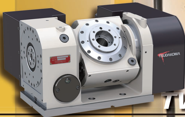
TWA-160
